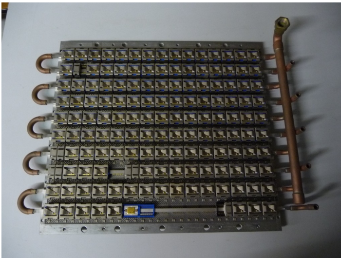
CDC Cyber 855 Modul (Freon gekühlt)
