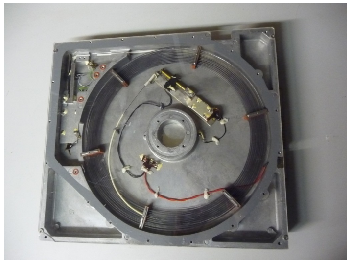
CDC Mechanische Delay Line eines Terminal Controllers
