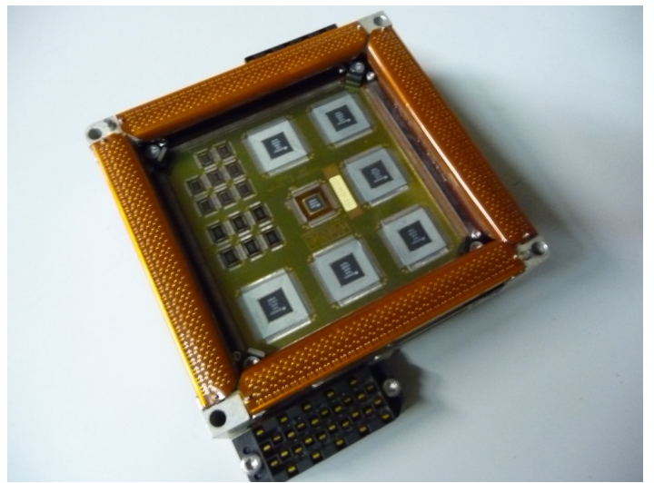
DEC VAX 9000 CPU Modul
