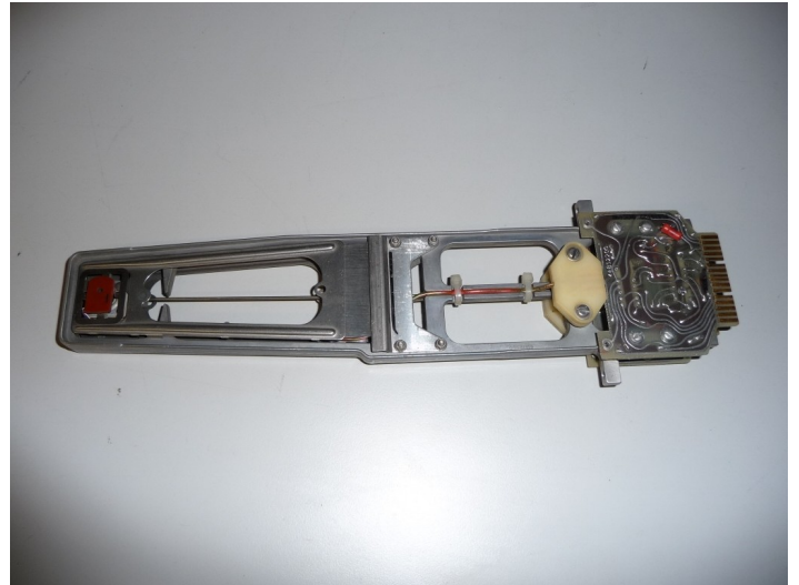
CDC 821 Disk Lese-/Schreibkopf
