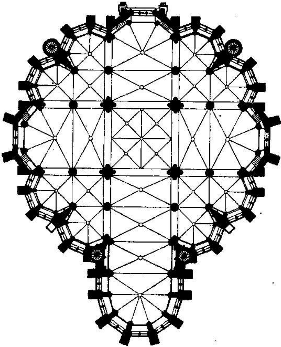
Trier, Liebfrauenkirche (1235–50) (Grundriss: Dehio/v. Bezold 1894)
