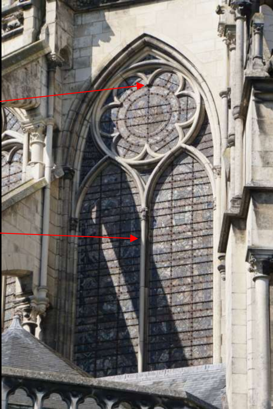
Masswerk, Begriffe (Beispiel Kathedrale von Troyes)
