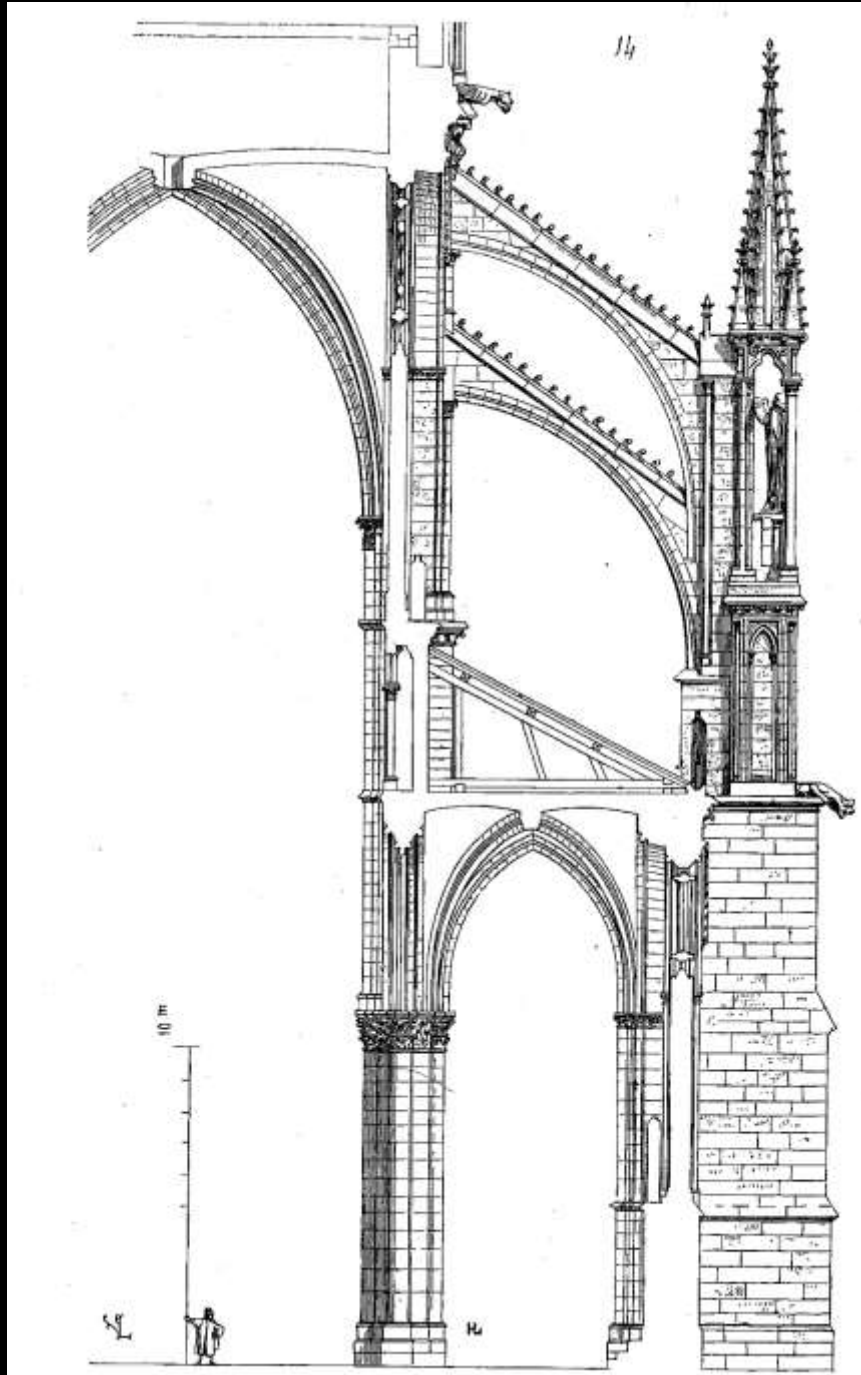
Reims, Kathedrale, Querschnitt des Langhauses (Viollet-le-Duc)
