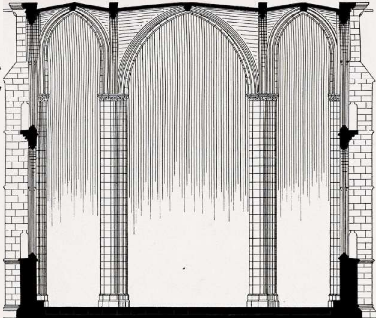
Marburg/Lahn, Elisabethenkirche (1236–86; Zeichn.: Dehio/v. Bezold 1894, bearb.). Raumform der Hallenkirche
