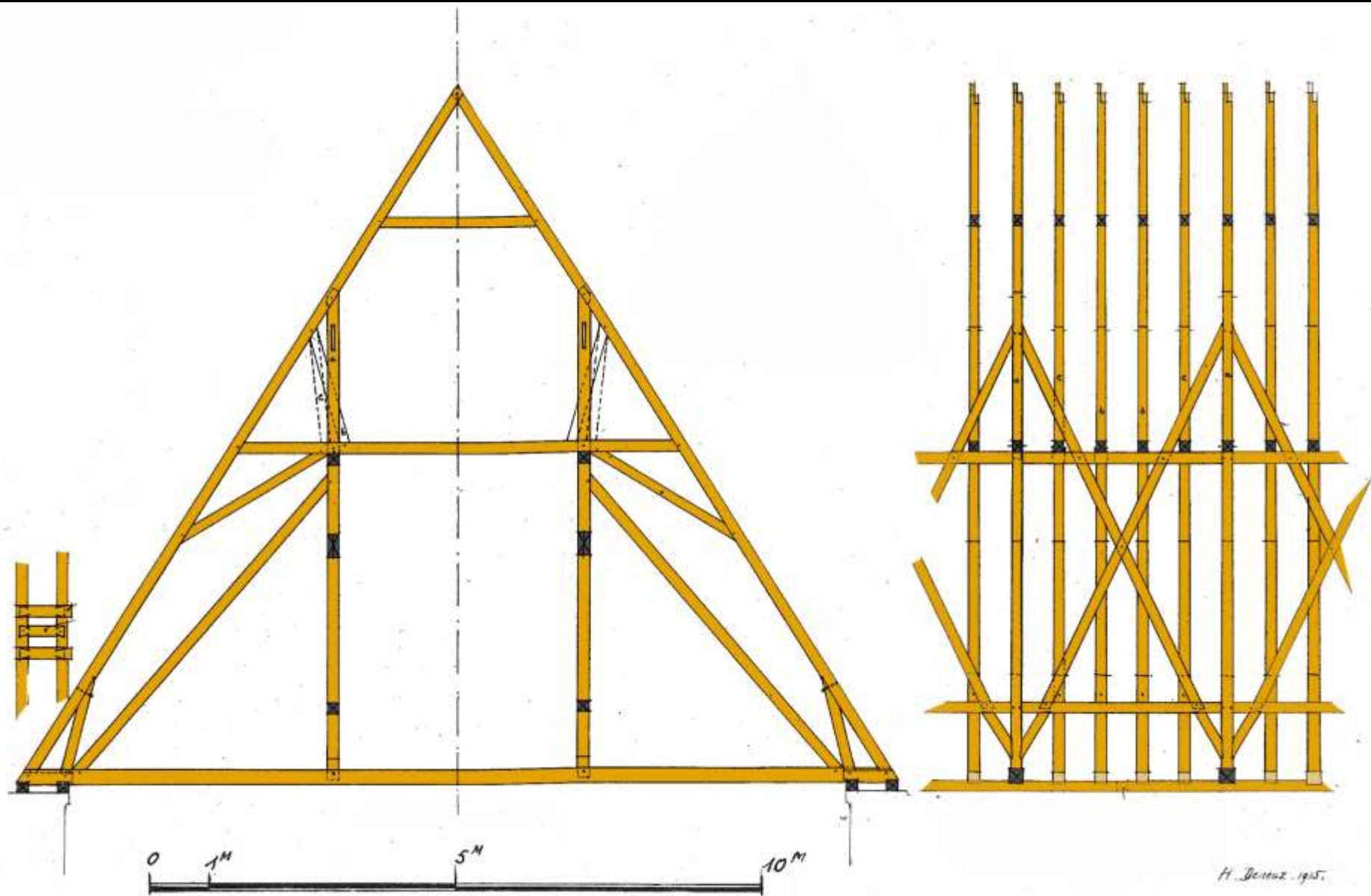
Auxerre, Kathedrale, Dachwerk über dem Chor mit „stehendem Stuhl“ (Baufaufnahme Henri Deneux 1915, bearb., aus CRMH 1972)
