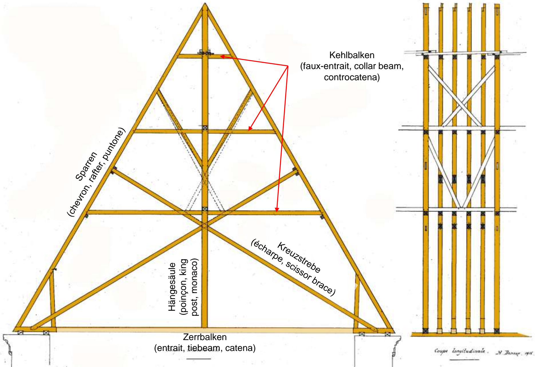
Sens, Kathedrale, Chor, Dach (Längsverband später hinzugefügt): reines Sparrendach (chevrons formant fermes) (Baufaufnahme von Henri Deneux 1916, bearb., aus CRMH 1972)
