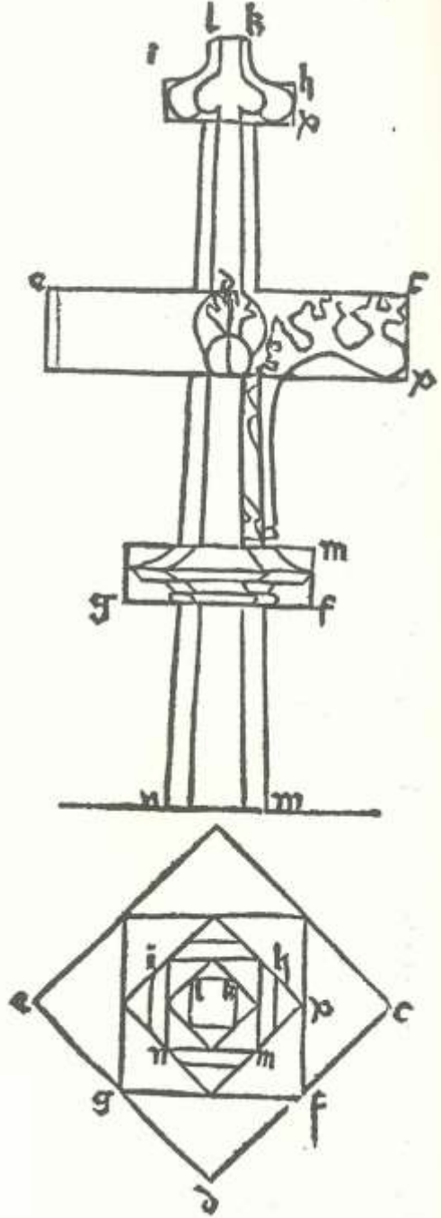
geometrische Konstruktion einer Kreuzblume
