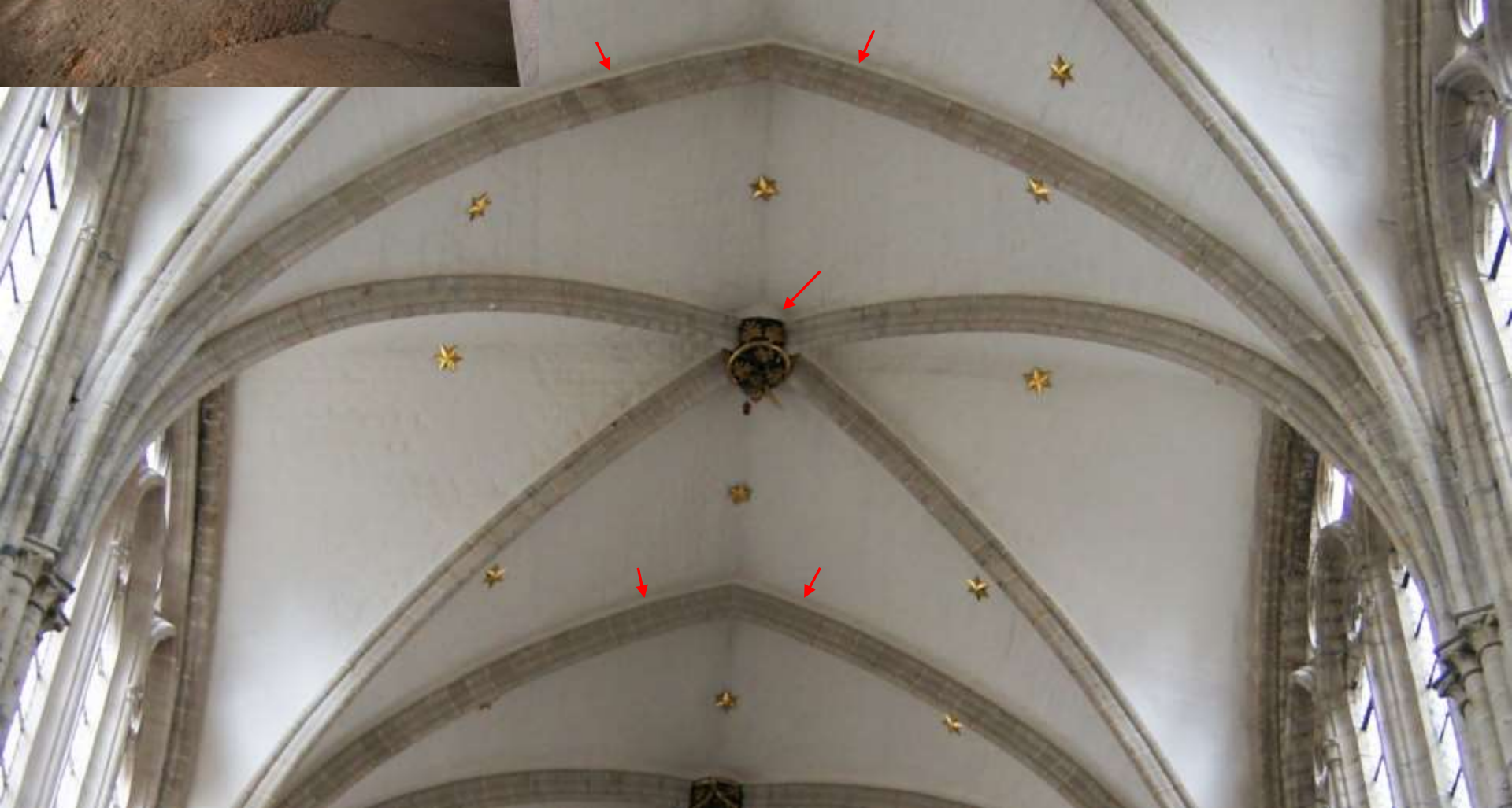
Kreuzrippengewölbe mit horiz. Scheitel, Brüssel, Saint-Michel-Sainte-Gudule, Langhaus, 14. Jh.
