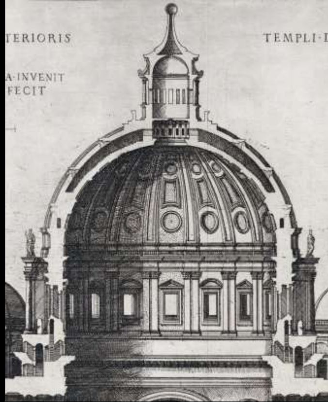
Michelangelo Buonarotti (1475–1564) und seine Pläne für St. Peter in Rom: Rückkehr zum Zentralbauprojekt und Idee der doppelschaligen Kuppel 1546–64
