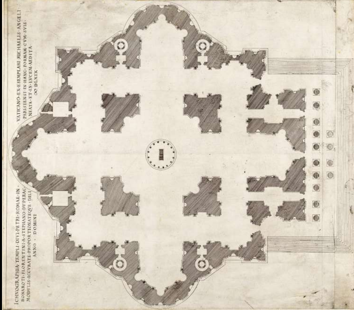
Rom, St. Peter, Plan Michelangelos (nach 1546) (Stich von E. Dupérac, 1569, Metropolitan Museum, New York)
