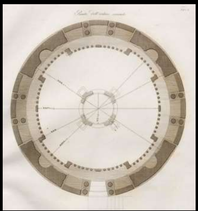
Verona, Cappella Pellegrini: Grundriss in Höhe Tambour und Schnitt, Vergleich zu Bramantes St. Peter (Zeichnungen: Serlio 1540/1600 und Sanmicheli/Giuliani 1816, ETH-Bibliothek)
