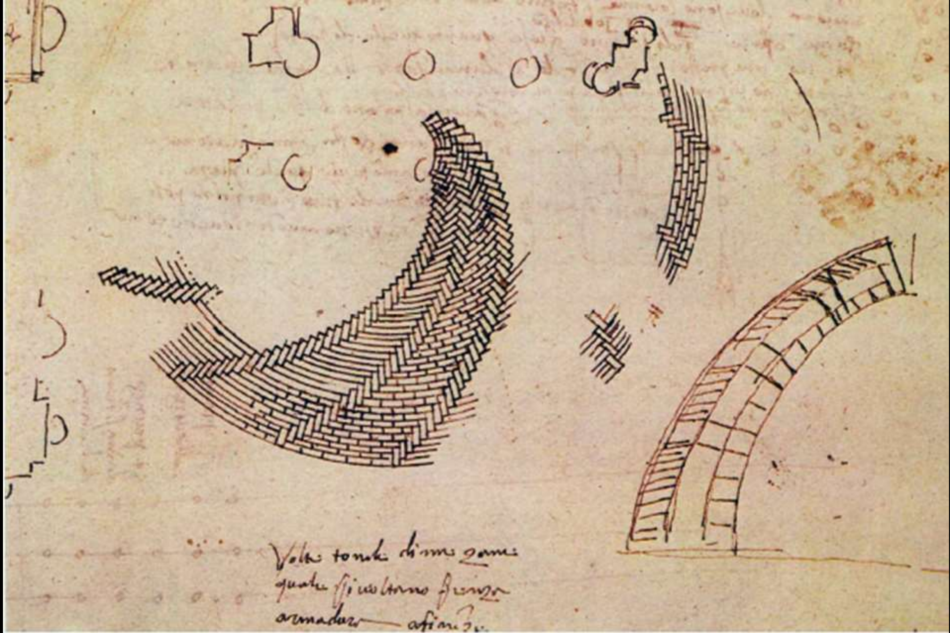
Antonio da Sangallo d. J. (um 1510): „Spinapesce“-Mauerwerksverband „volta tonda di mezza gamba quale si voltano senza armatura a Firenze“ (Uffizien, Florenz, GDSU 900 A).
