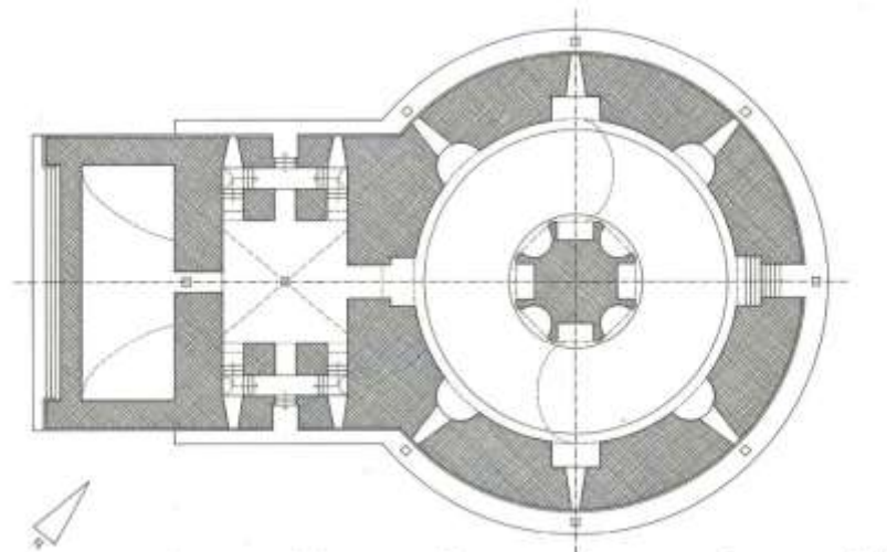
A Fundamentplan (Schnittebene in Höhe des Entwässerungskanal)
