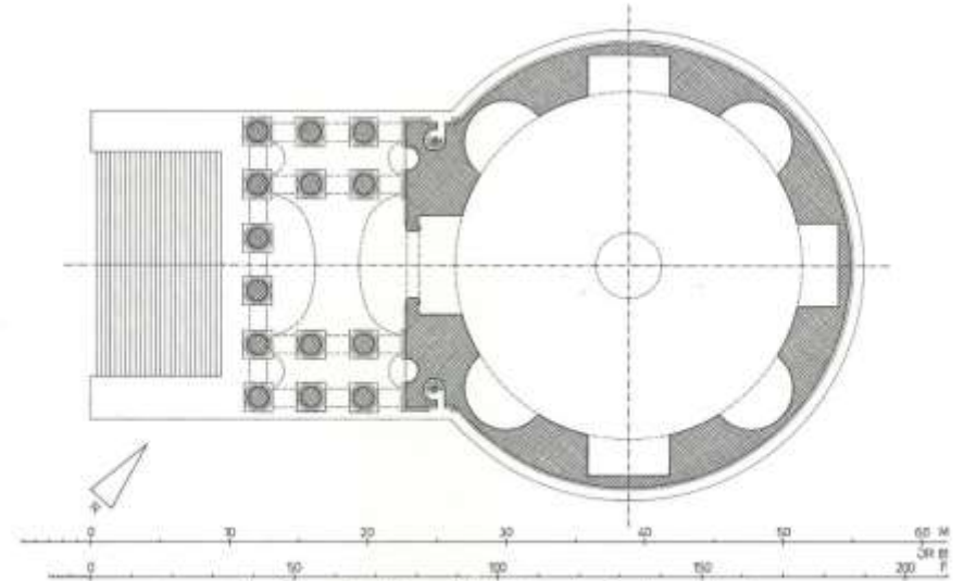
A Obergeschoß-Grundriß (nicht in allen Details gesichert)
