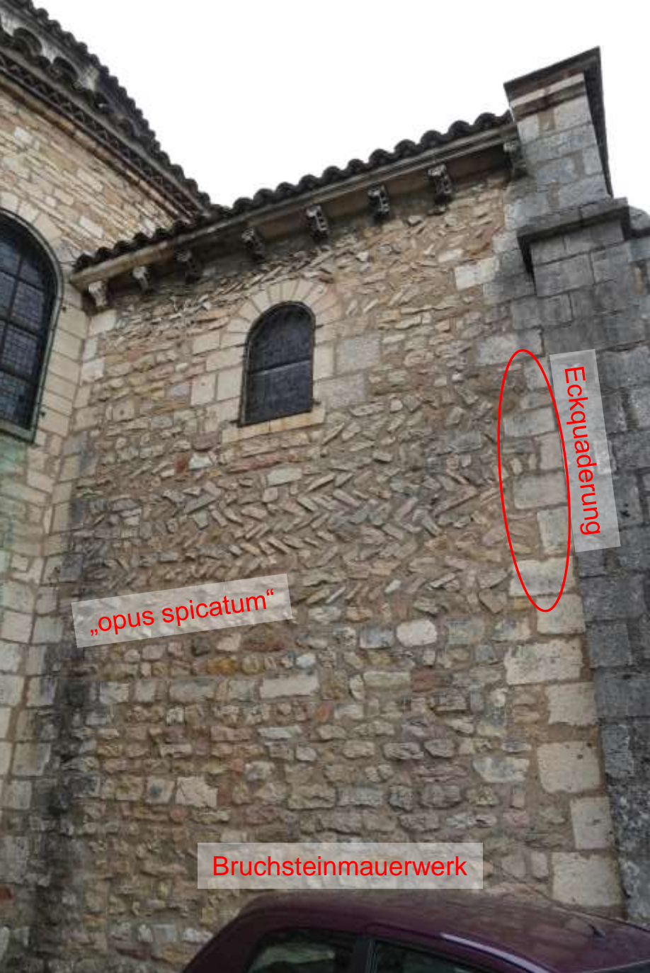
Tournus, Saint-Philibert. Bruchsteinmauerwerk (um 1008) an einer Radialkapelle des Chorumgangs
