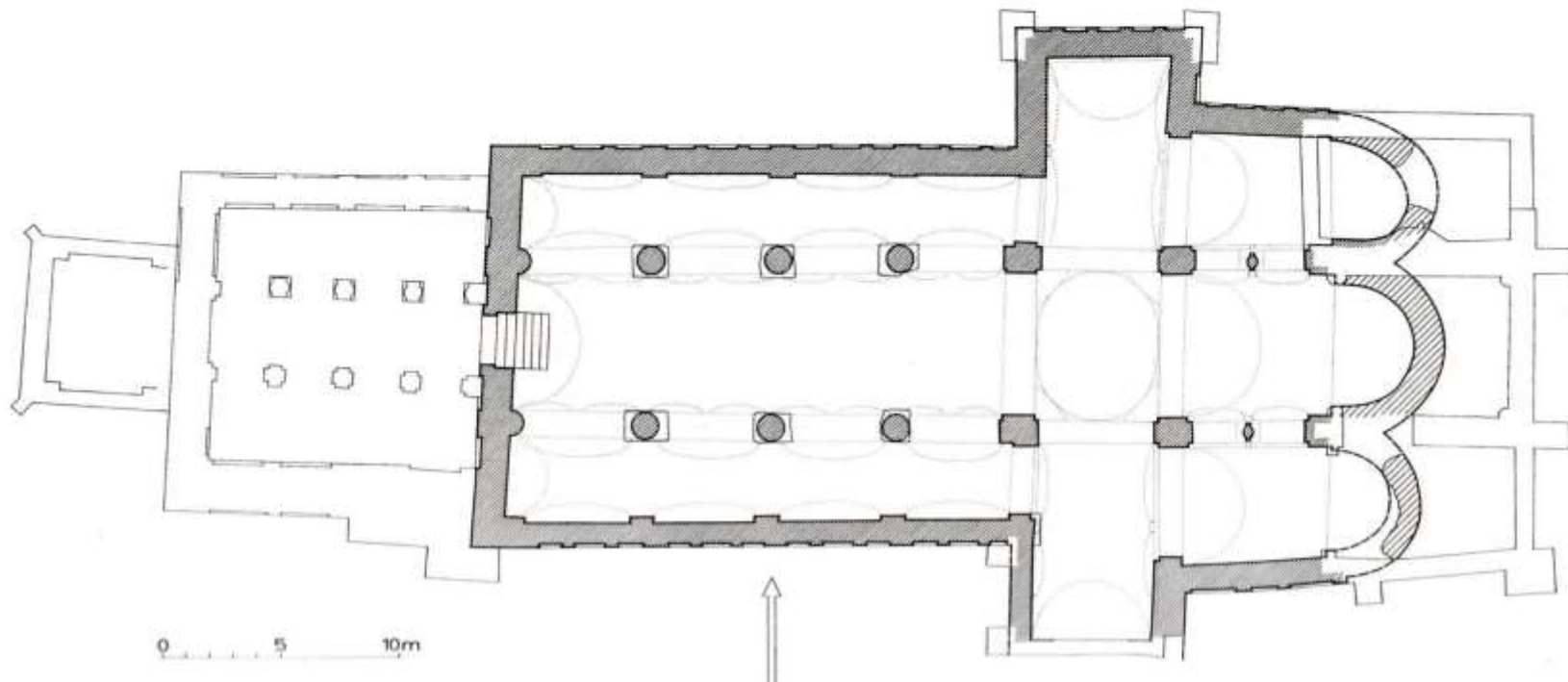
Romainmôtier, Abteikirche (Rekonstruktion des Zustandes um 1100; Sennhauser 1970)
