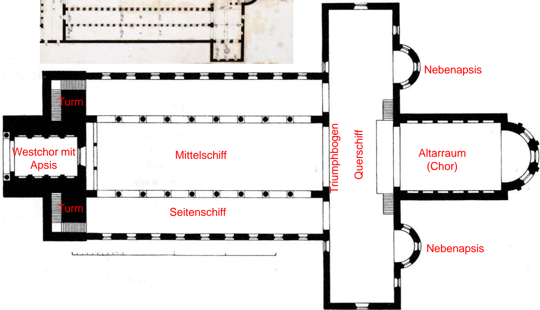
Bad Hersfeld, Stiftskirche, Mitte 11. Jh. Grundriss (Dehio/v. Bezold)
