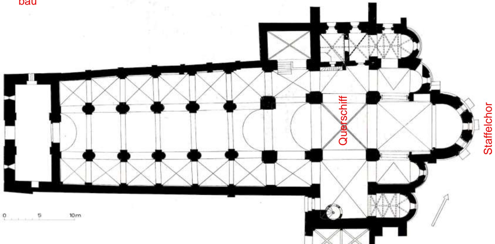
Payerne (VD), Abteikirche, spätes 11. Jh. Grundriss (Sennhauser 1970)
