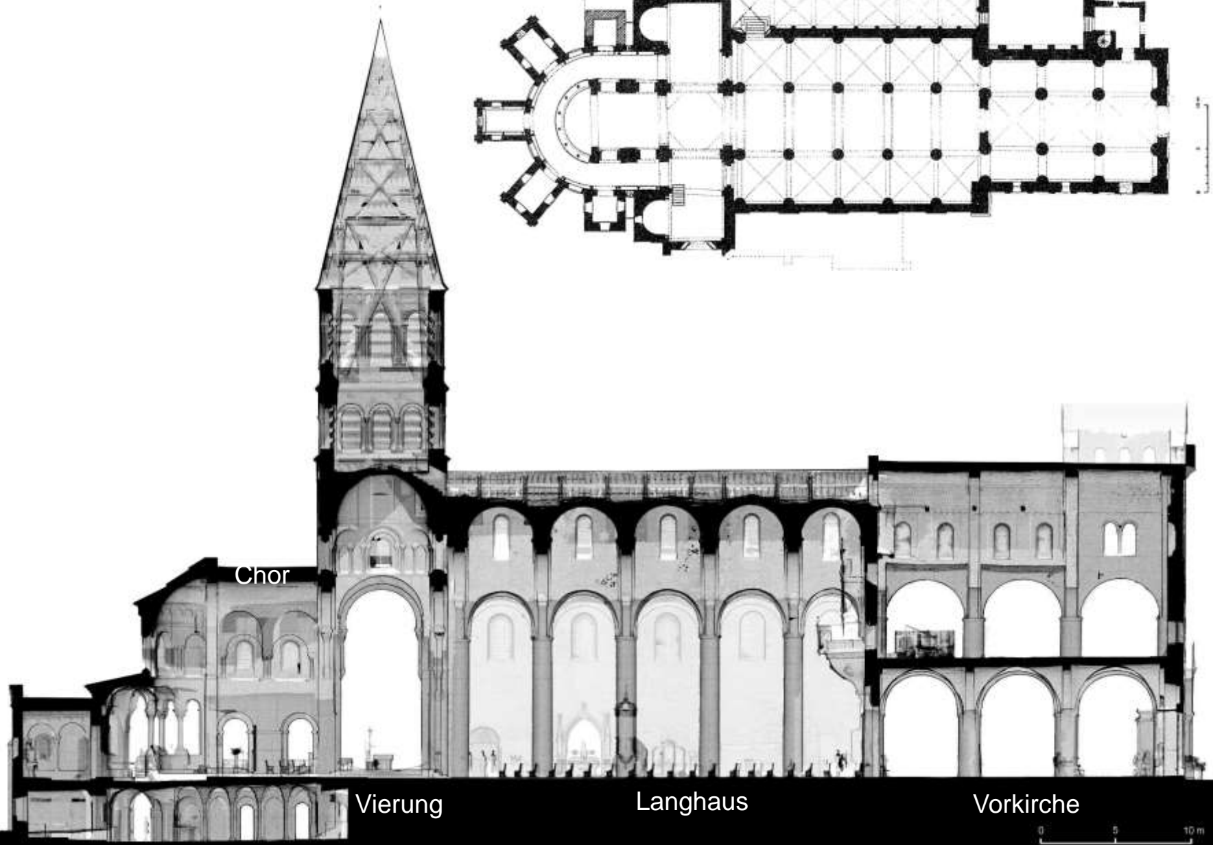
Tournus, Saint-Philibert. Längsschnitt (Scan: IDB, ETH Zürich, 2021)
