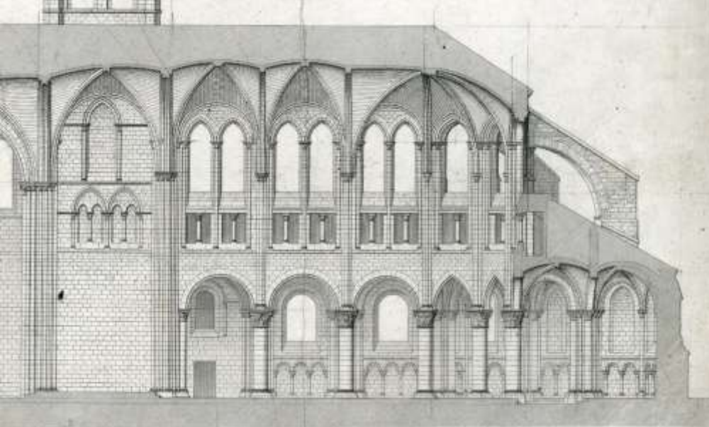
(Baufaufnahme: Lenoir 1867)
