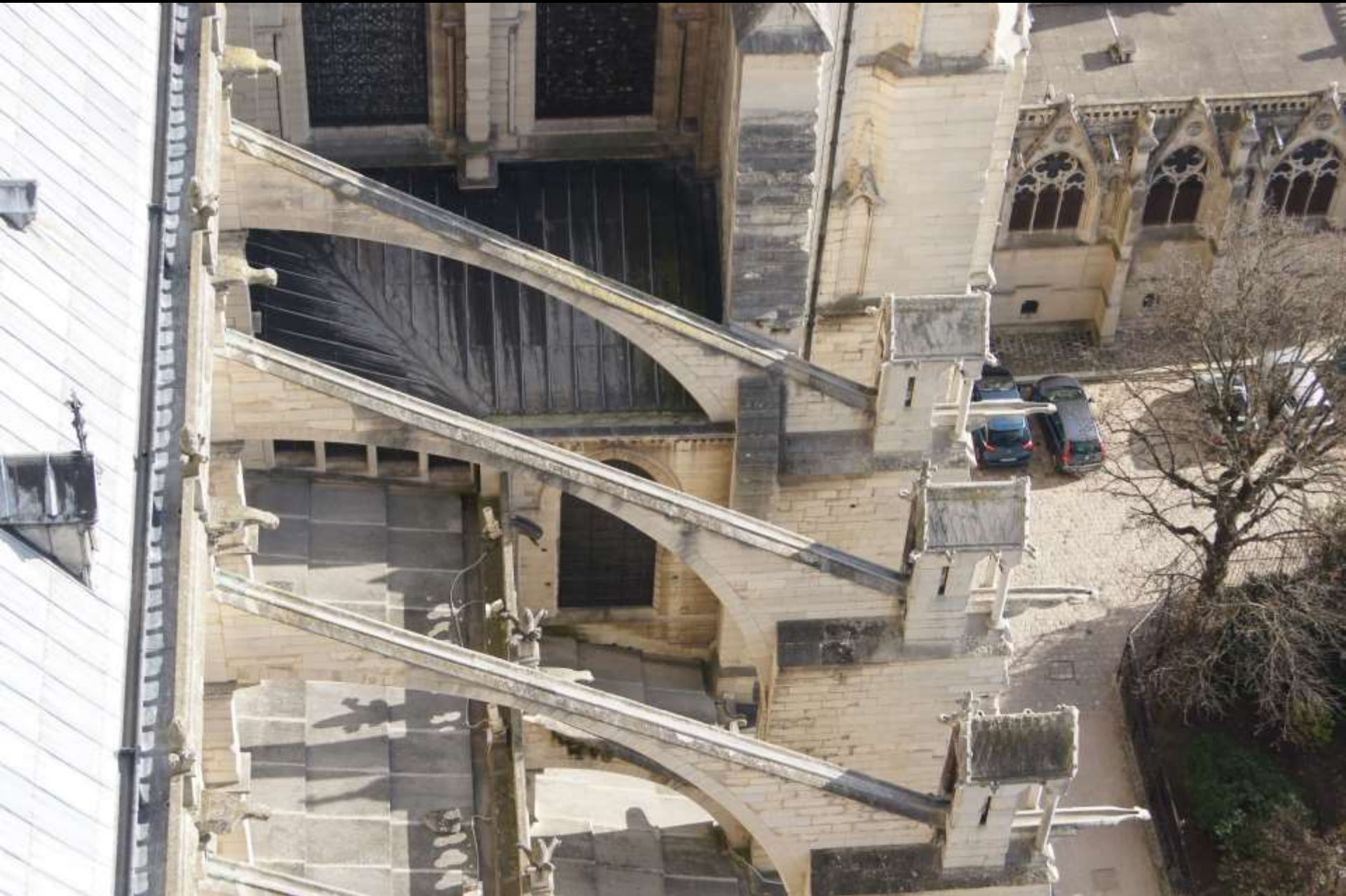
Paris, Kathedrale Notre-Dame, heutiges Strebewerk am Langhaus (14. Jh., erneuert 19. Jh.)
