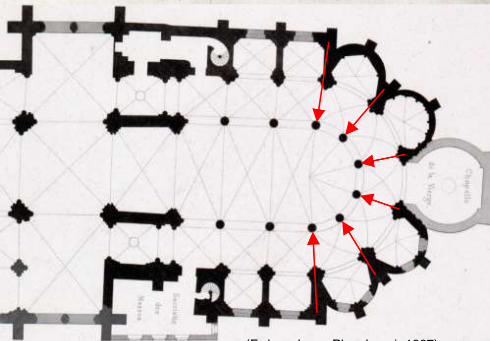
(Erdgeschoss, Plan: Lenoir 1867)
