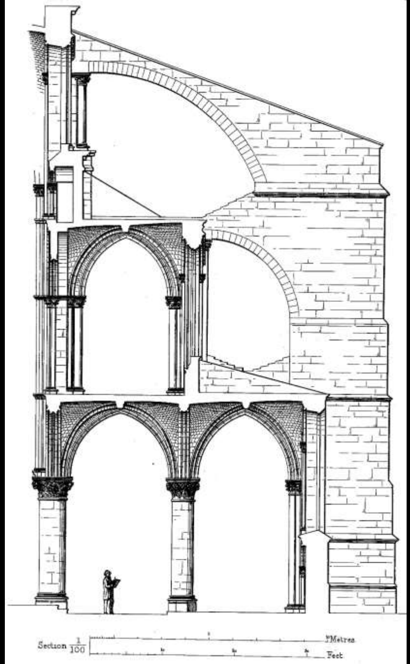
Zum Vergleich: Strebewerk der Abteikirche Saint-Remi in Reims, um 1170 (King 1858)
