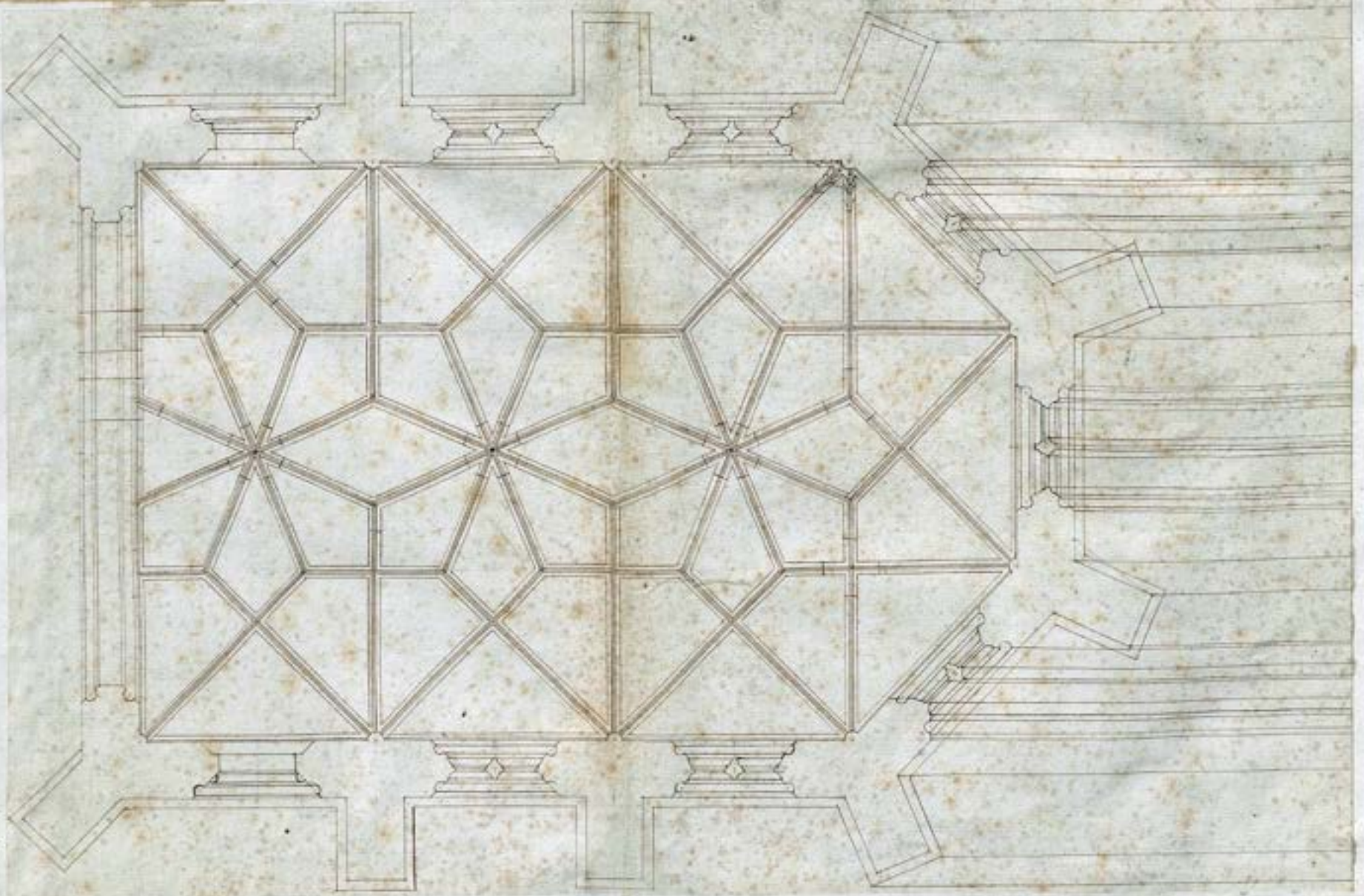
Gotisches Lehrbeispiel für ein Rautennetzgewölbe (Württ. Landesbibl. Stuttgart, Slg. Nicolai, Bd. 5)
