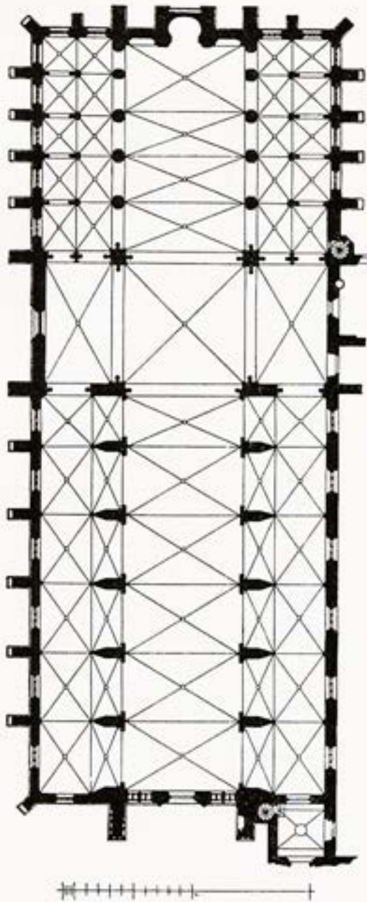
Salem, Abteikirche (1299 – um 1325). Grundriss (Dehio/v. Bezold 1894) und Inneres.
