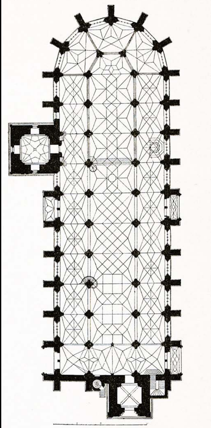
Dinkelsbühl, St. Georg (2. H. 15. Jh.). Grundriss (Dehio/v. Bezold 1894) und Langhausgewölbe
