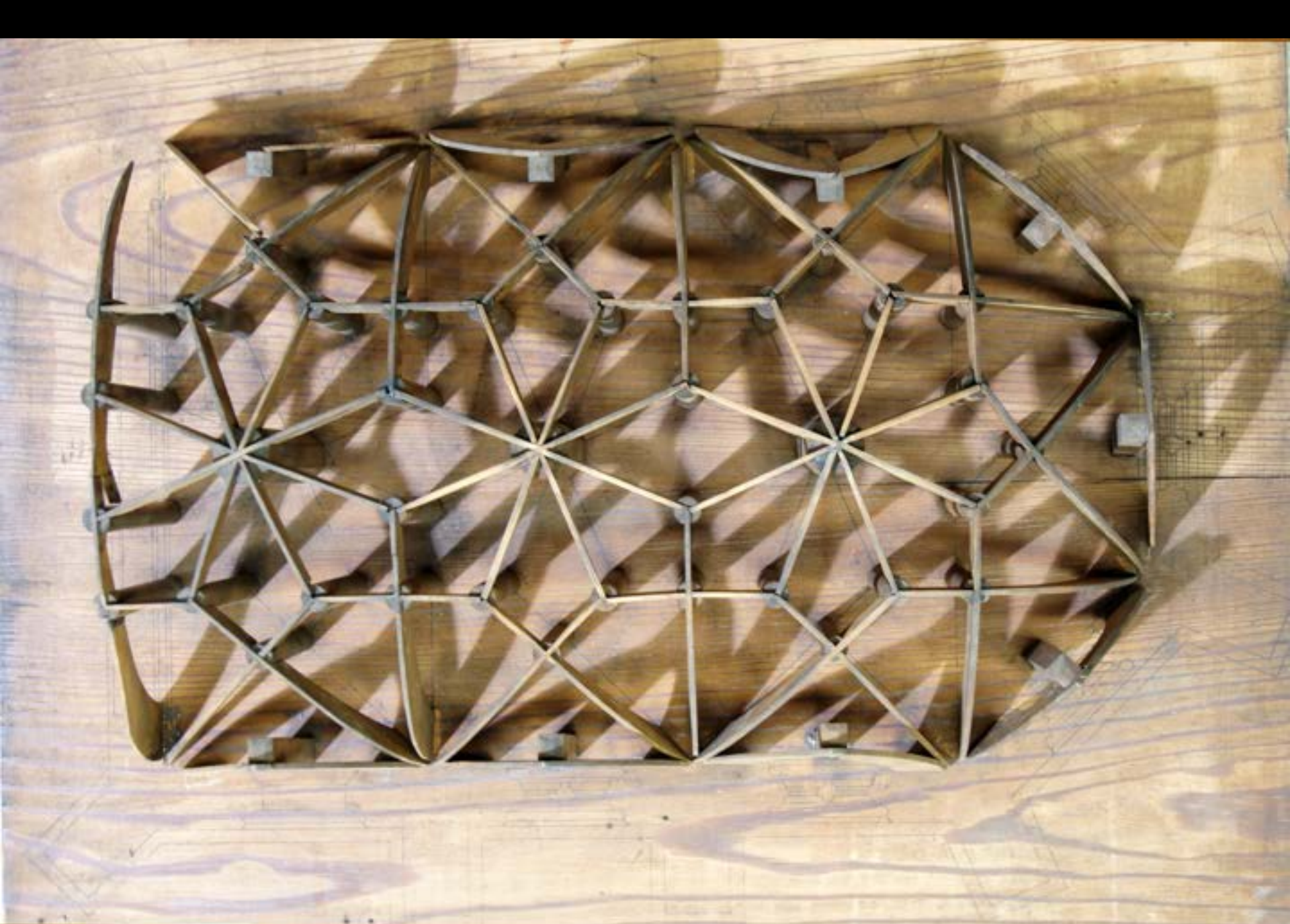
Gotisches Lehrbeispiel für ein Rautennetzgewölbe (Bamberg, Städt. Museen)
