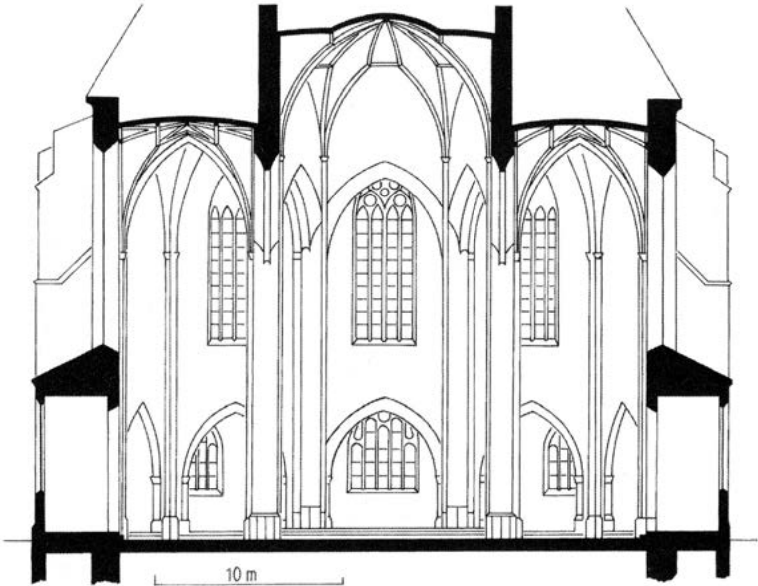
Ingolstadt, Liebfrauenkirche (1425 – Anf. 16. Jh.) (Schnitt: Ingolstadt 2002)
