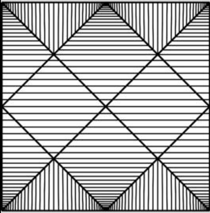
Parallelrippen-Netzgewölbe als elliptische Tonne mit Stichkappen
