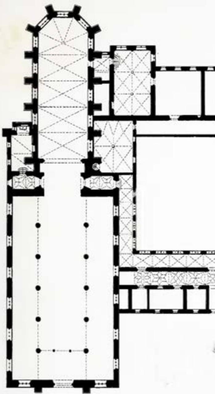
Regensburg, ehem. Franziskanerkirche (Minoritenkirche), 2. H. 13. Jh. und Mitte 14. Jh. (Grundriss: T.H. King 1858, bearb.)
