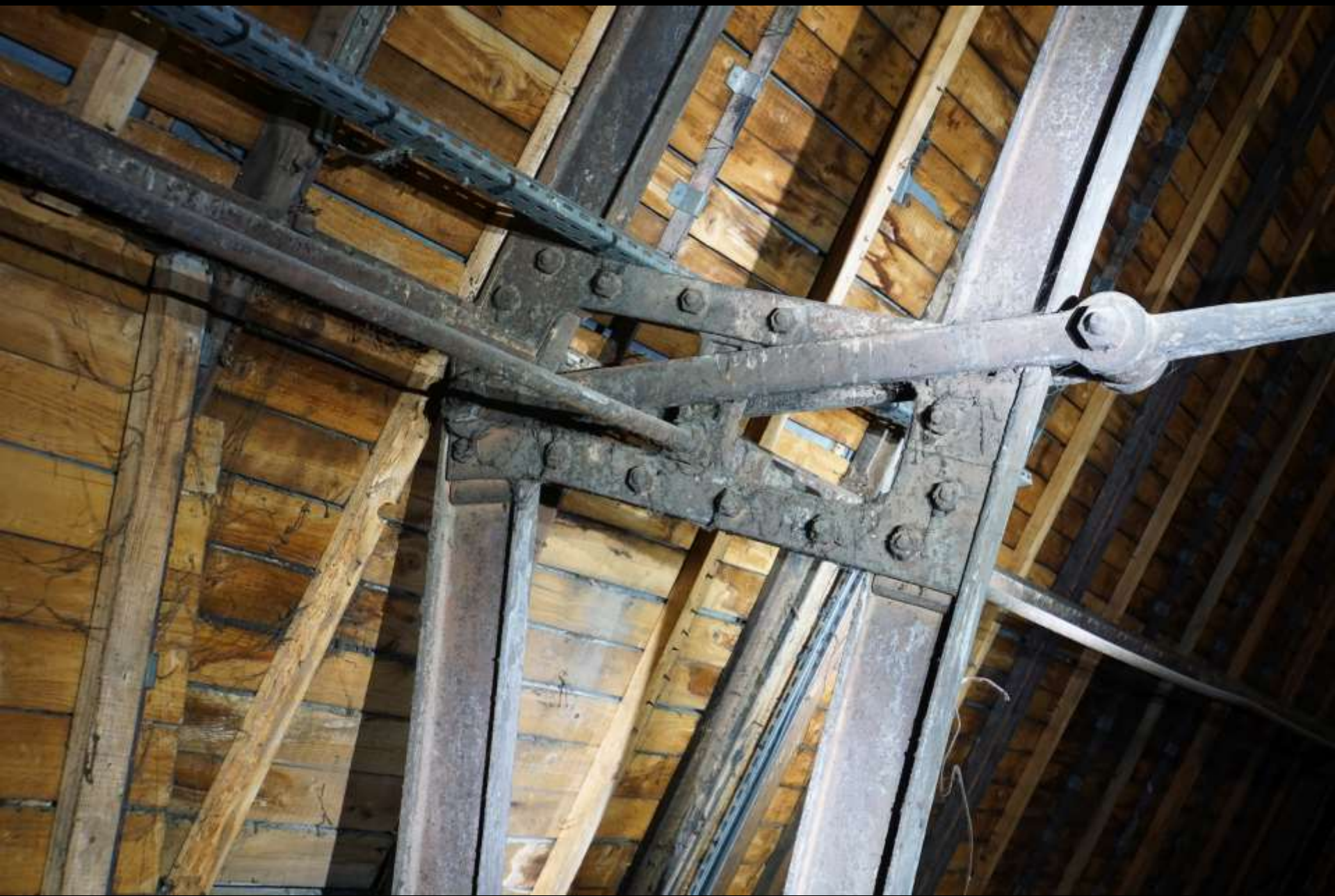
Paris, Sainte-Clotilde (Franz Christian Gau 1846-57). Anschlüsse mit Sechskantschrauben
