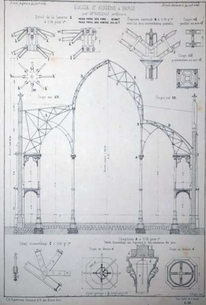
Paris, Saint Eugène (Louis Auguste Boileau, 1855). Versteckte Konstruktion aus Schmiedeeisen. (Nouvelles Annales de la Construction, 1856)
