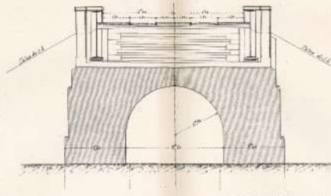
Fig. 6. Coupe d'une pile à 0 01 pour 1 m .
