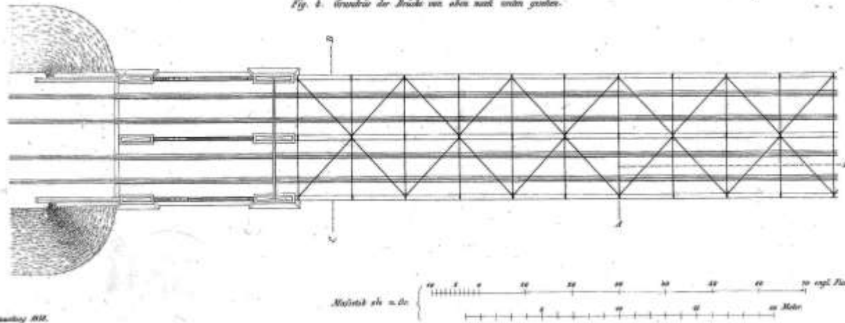
Fig. 4. Grundriß der Brücke von oben nach unten gesehen.
