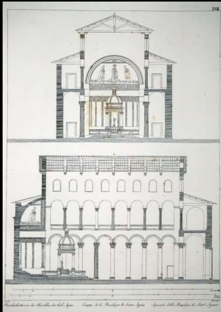
Rom, Sant' Agnese fuori le mura, 7. Jh. Grundrisse und Schnitte (Gutensohn/Knapp 1822-27) Emporenbasilika
