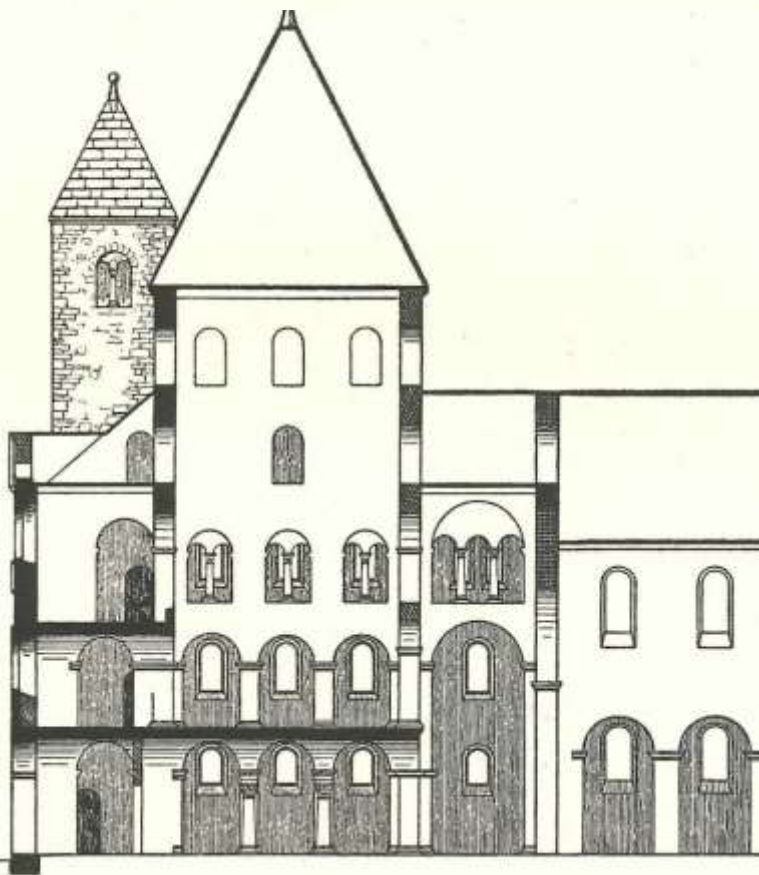
Corvey, Abteikirche, Westwerk (Rekonstruktion des Zustandes 885: Effmann 1929)
