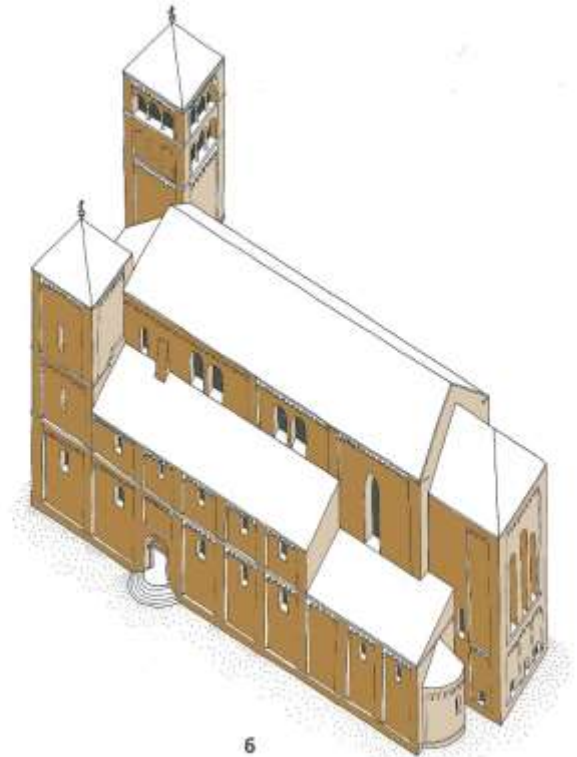
Zürich, bauliche Entwicklung des Grossmünsters (Gutscher 1983)
