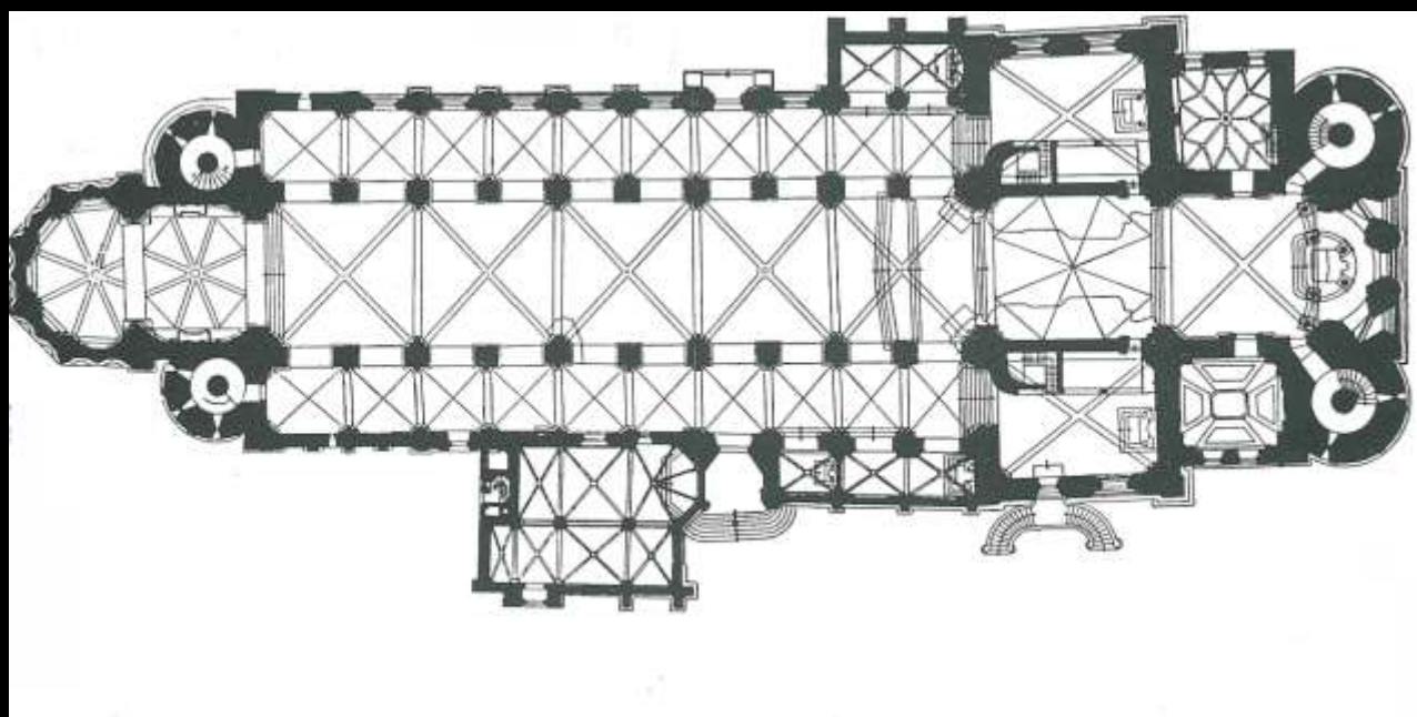
Worms, Dom (1125 – nach 1185)
