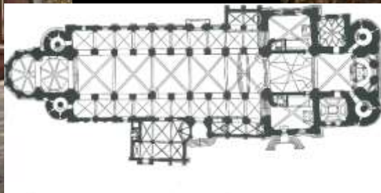
Worms, Dom (1125 – nach 1185). West- und Ostchor
