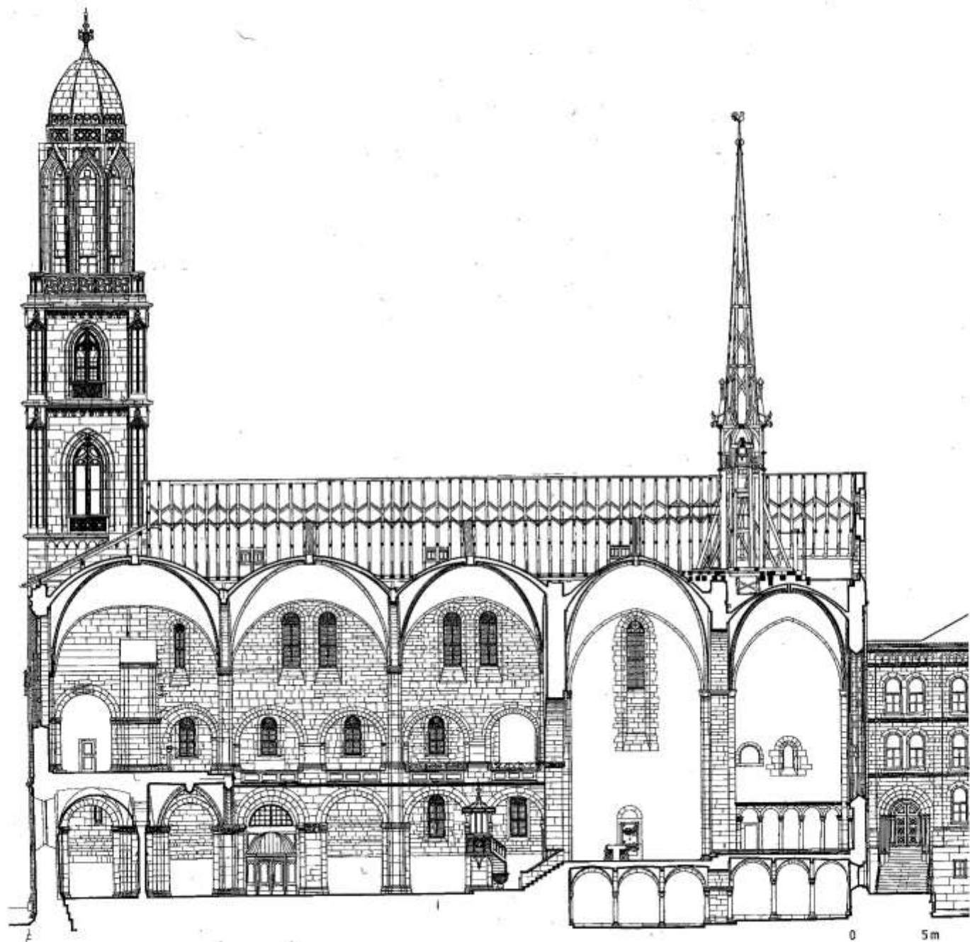
Zürich, Grossmünster, Längsschnitt (Gutscher 1983)
