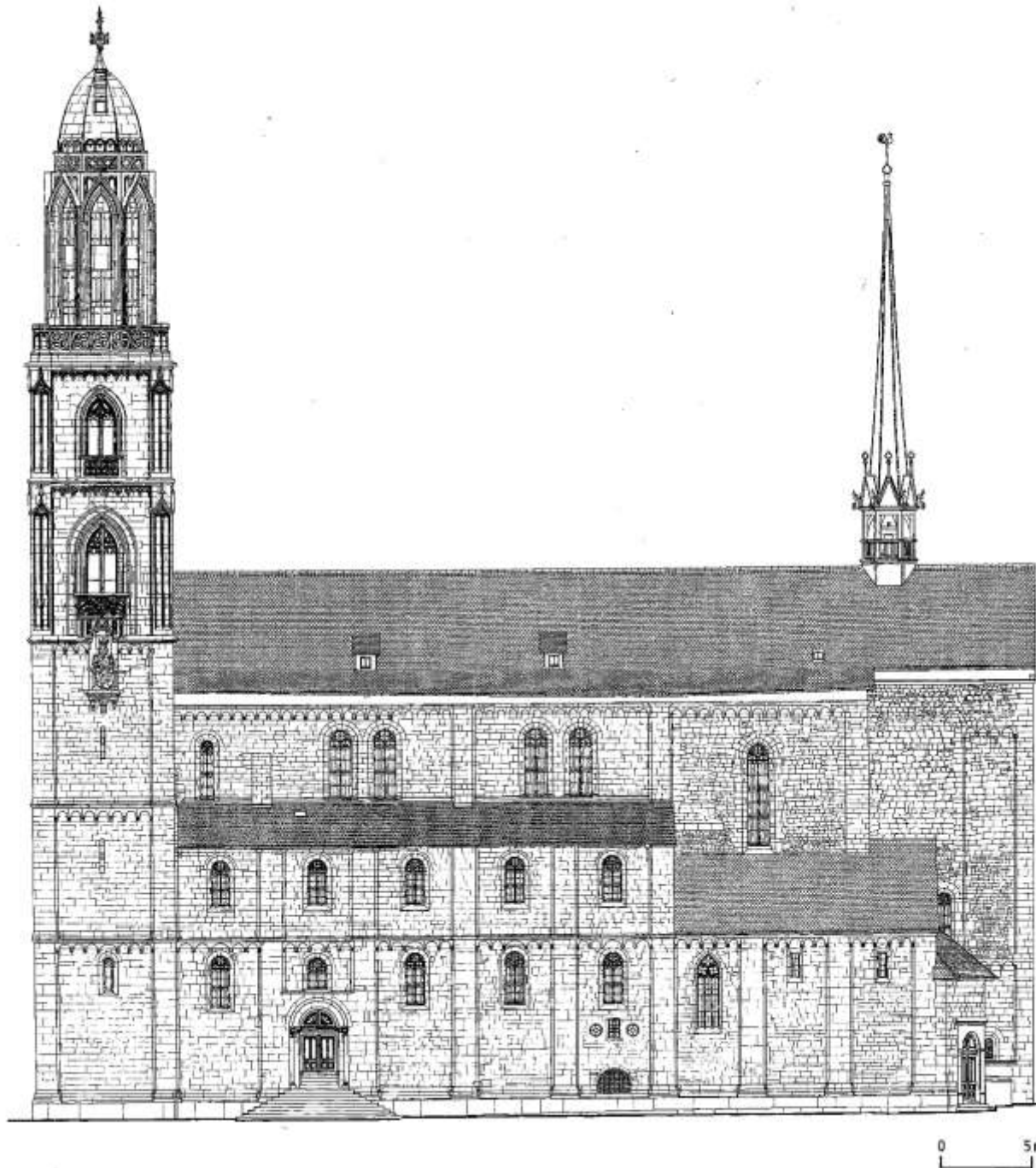
Zürich, Grossmünster, Südseite (Gutscher 1983)
