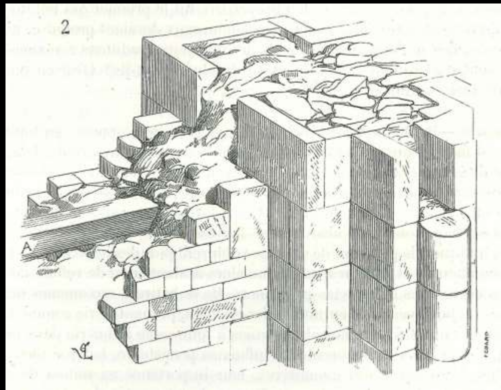
Cluny III, Konstruktion der Wand und der Wandgliederung (Zeichnung: Viollet-le-Duc)
