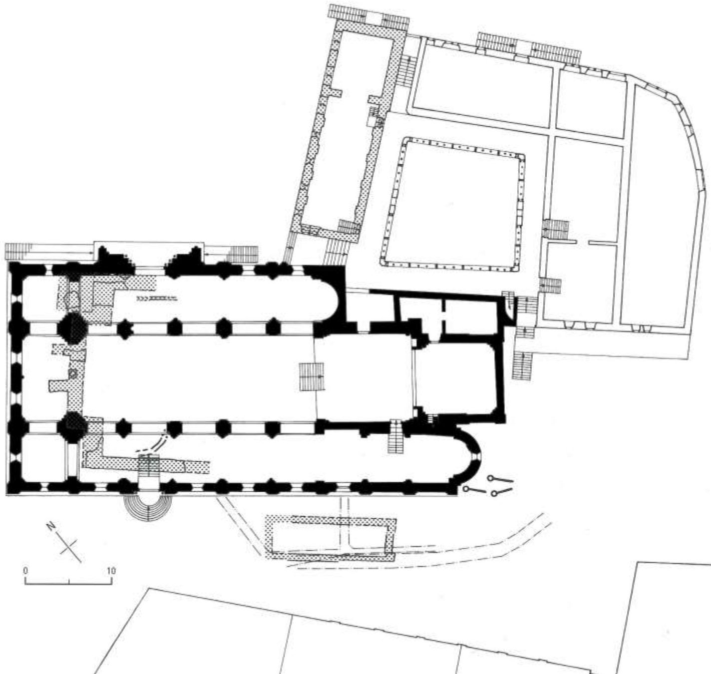
Zürich, Lageplan des Grossmünsters mit zugehörigem Kloster (Gutscher 1983)
