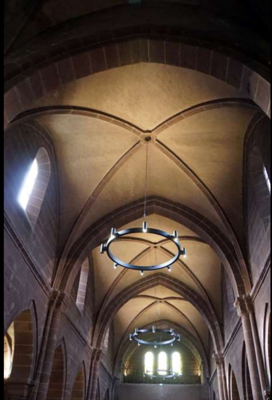
Gebweiler (Elsass), St. Leodegar (ca. 1180–1200)
