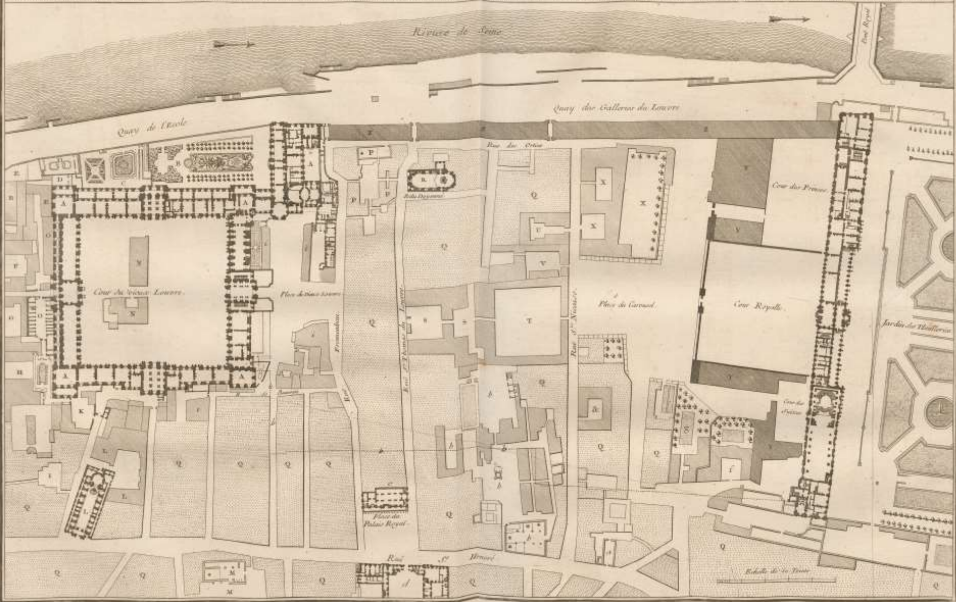
Plan General, au Rez de Chaussée de la disposition actuelle des Bâtimens du Louvre & du Palais des Thuilleries avec la Distribution des rues & les mailles des Maisons particulieres qui séparent ces deux Grands Edifices
