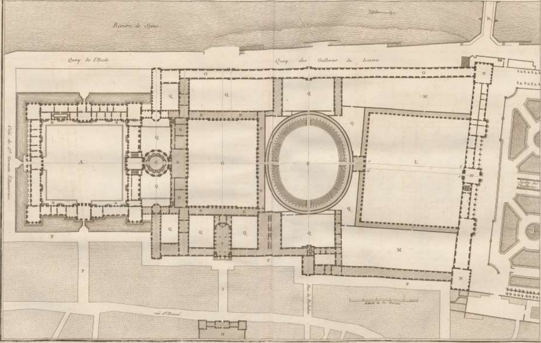
Erstes Gesamtprojekt von Claude Perrault, 1668 (in: Blondel, 1756)
