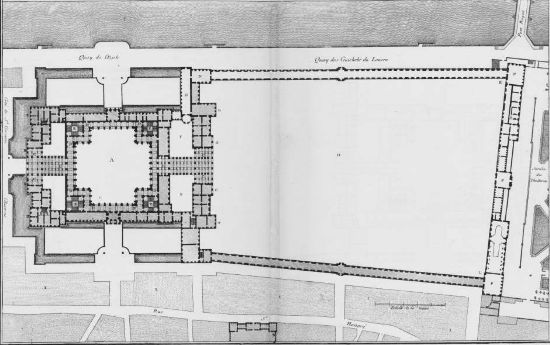
Berninis drittes Louvre-Projekt, 1665 (Stich von Marot)
