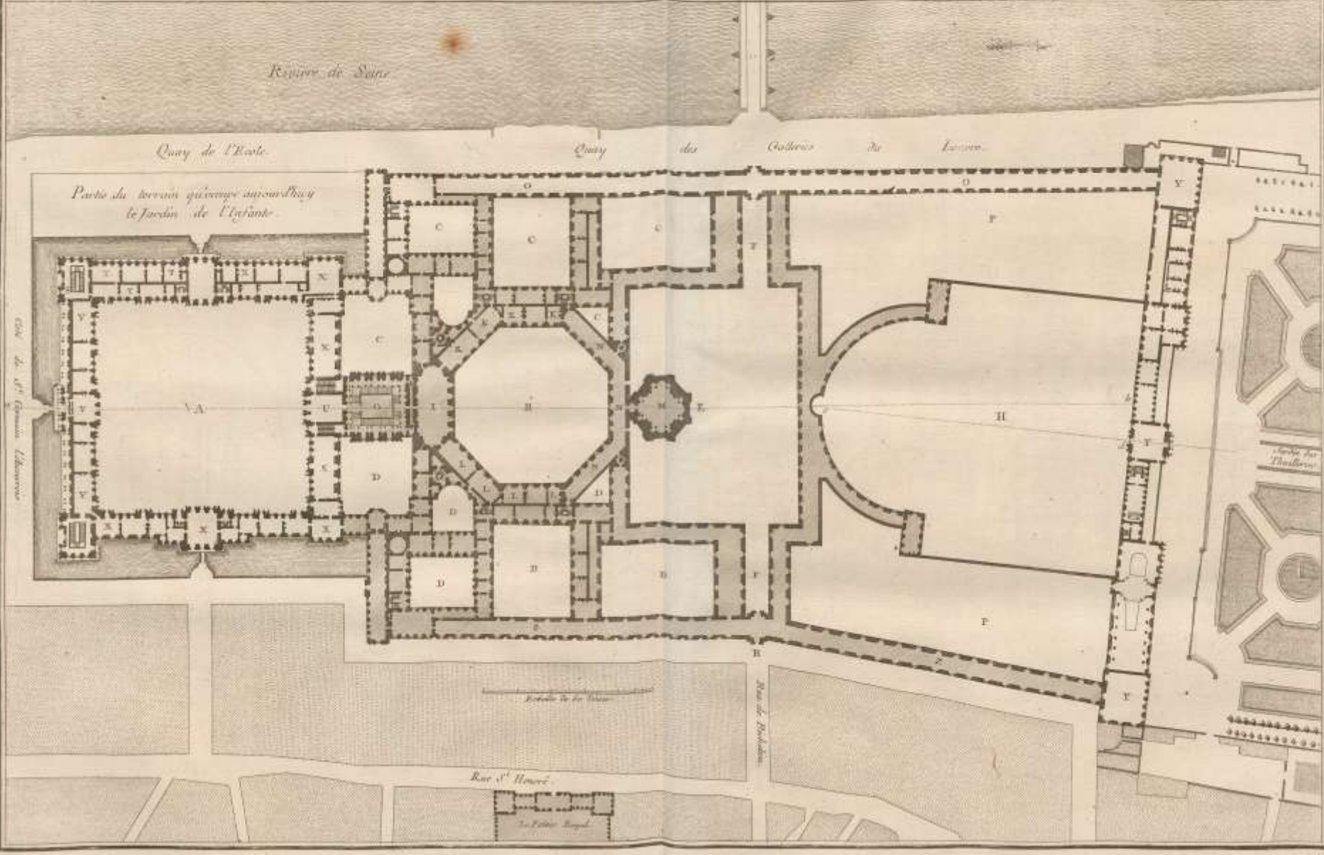
Zweites Gesamtprojekt von Claude Perrault, 1668 (in: Blondel, 1756)
