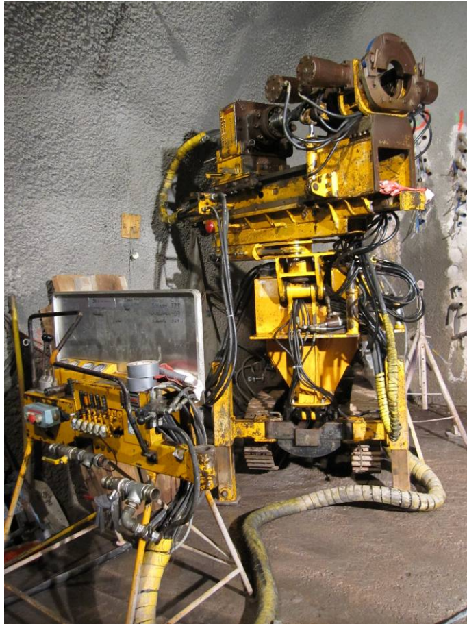
Bild 9: Bohrgerät Hütte 202 HBR
