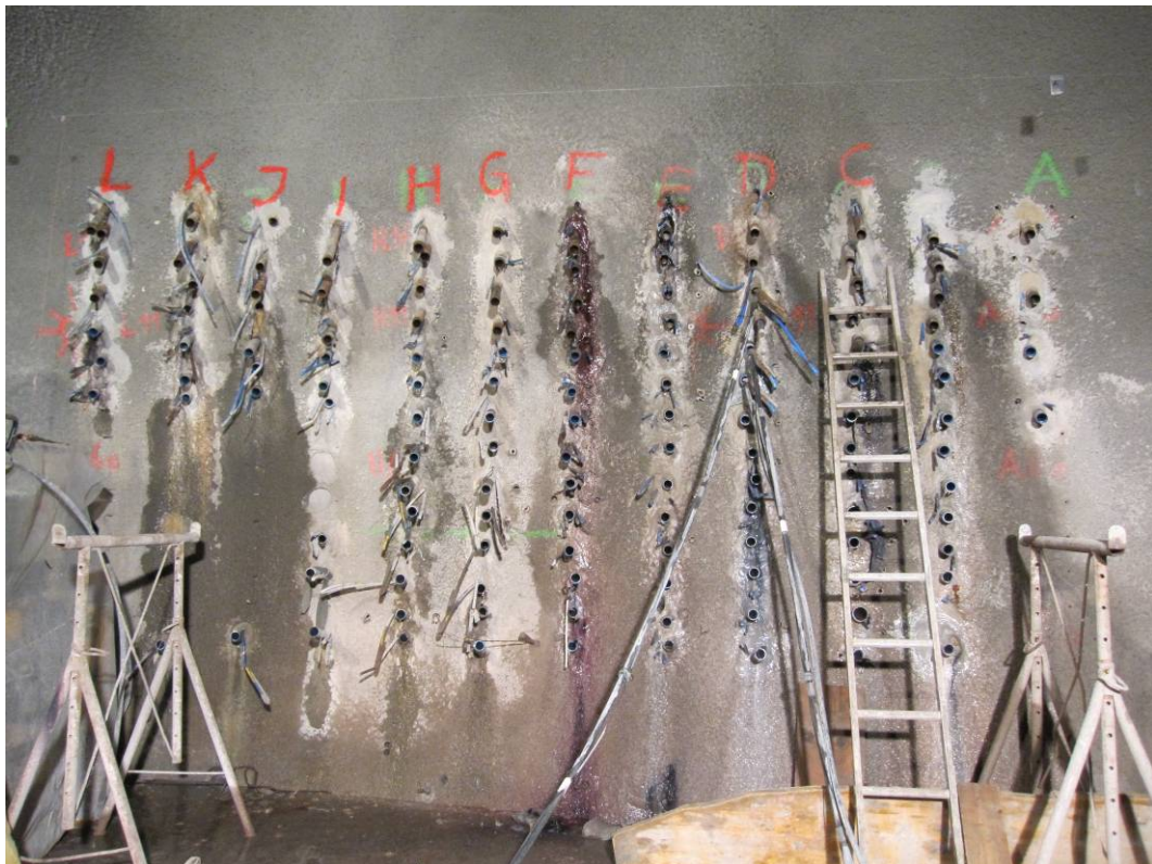
Bild 10: Ortsbrust mit vollzählig eingebauten Manschettenrohren; Injektionsnische
