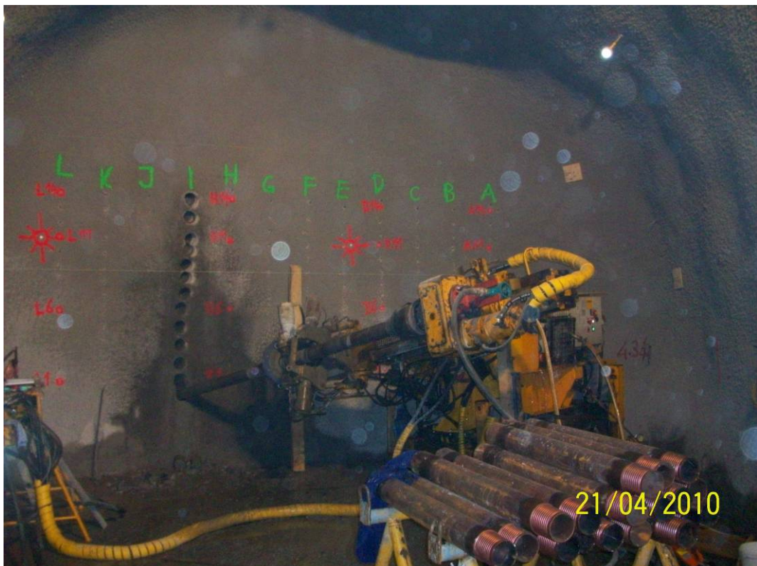
Bild 2: Bohrgerät Hütte 202 HBR während den Bohrarbeiten; Injektionsnische
