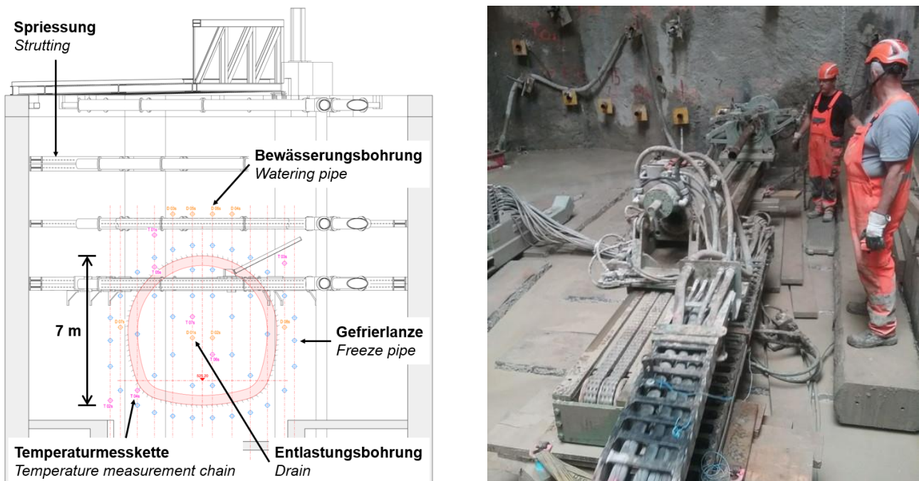
Bild 10: Stollen Laupenstrasse – links: Layout der Gefriermassnahme (Querschnitt, Blick in Vortriebsrichtung) [10]; rechts: Bohrarbeiten für die Gefriermassnahme [9]
