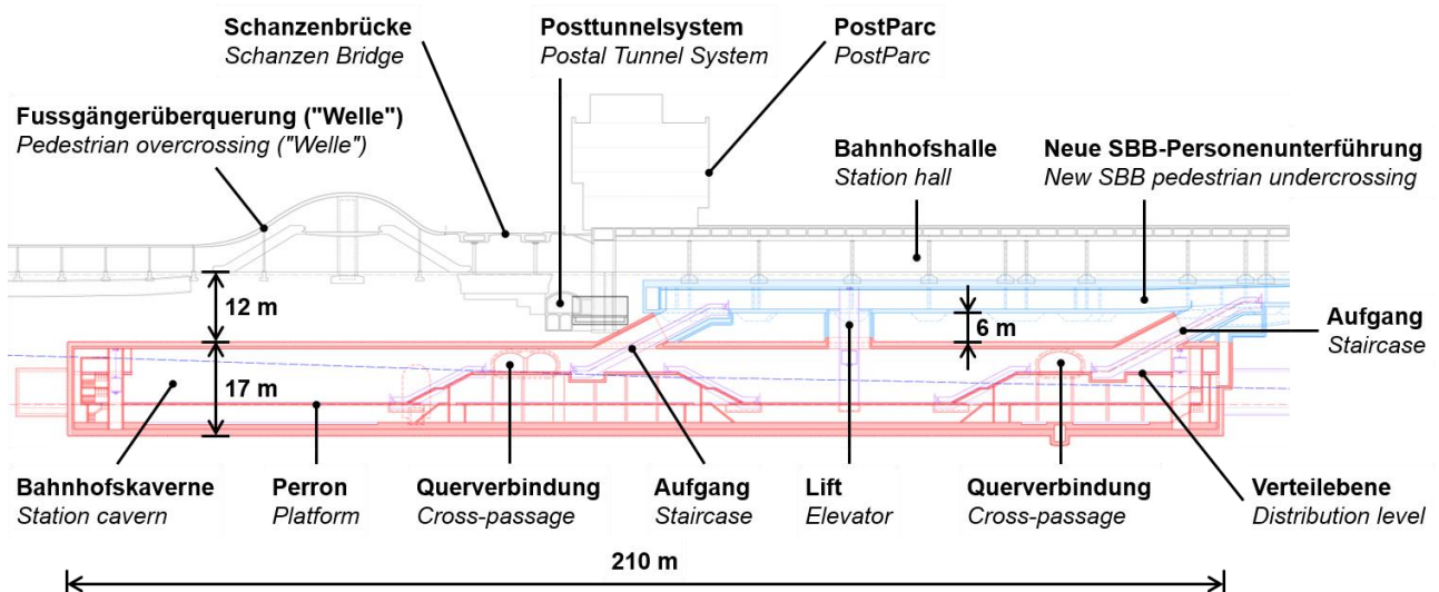
Bild 3: Bahnhofskavernen – oben: Situation; unten: Längsschnitt [6]
