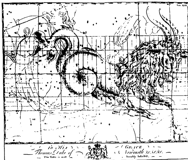
Fig. 25 - Il Capricorno, dall'Atlante Celeste di John Bevis, 1786.
