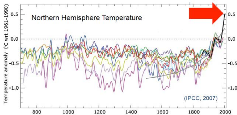
Abbildung 8: Paläo-Rekonstruktionen der Nordhemisphäre über die letzten 1000 Jahre (IPCC 2007d).
