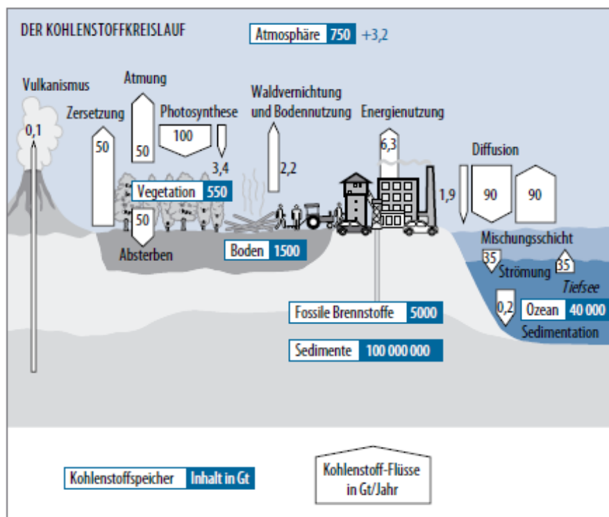
Abbildung 5: Der Kohlenstoffkreislauf [Gt C pro Jahr] (Liedtke, Welfens et al. 2008).
