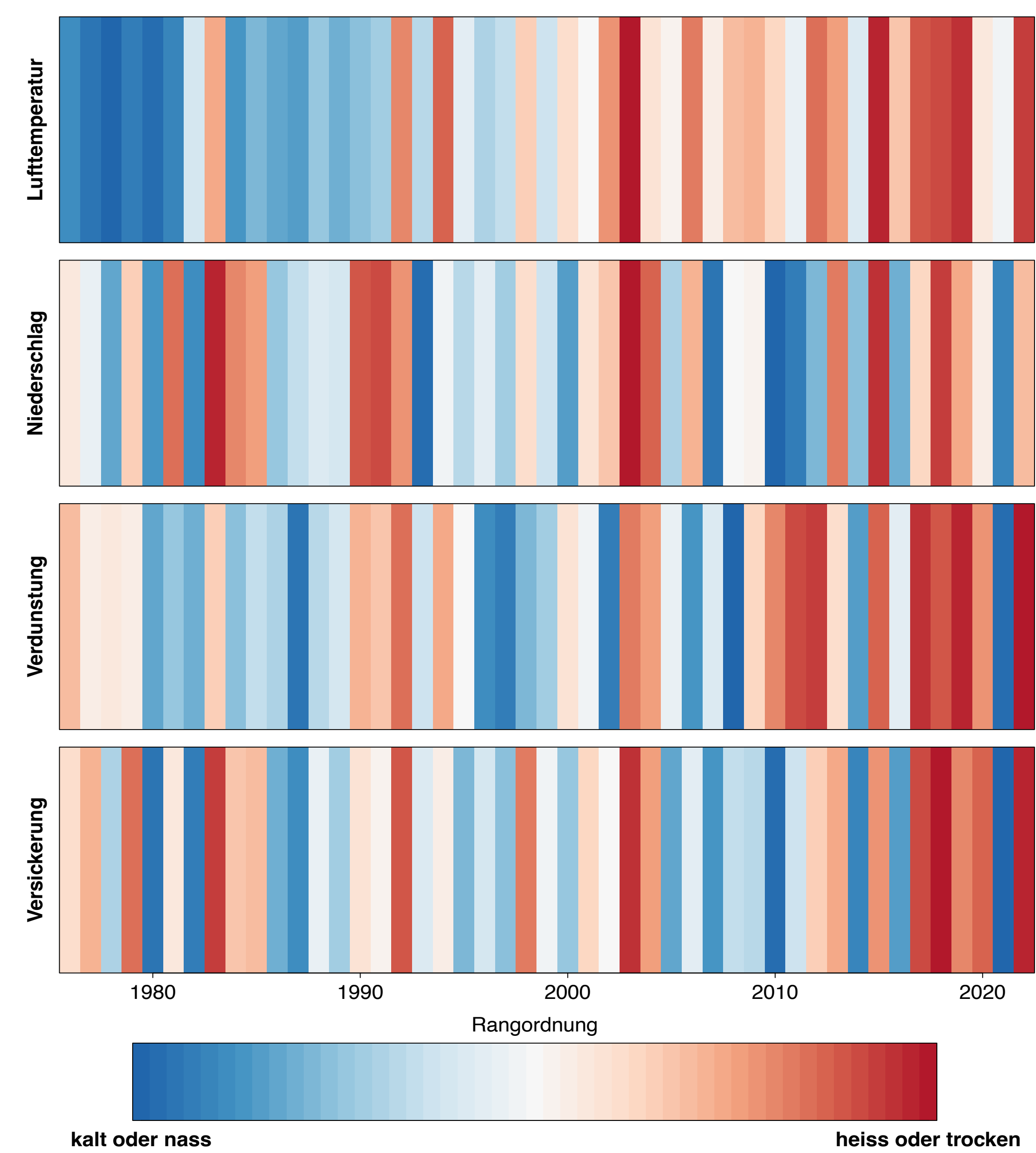
Rangordnung der heissen und trockenen Sommer am oberen Rietholzbach
